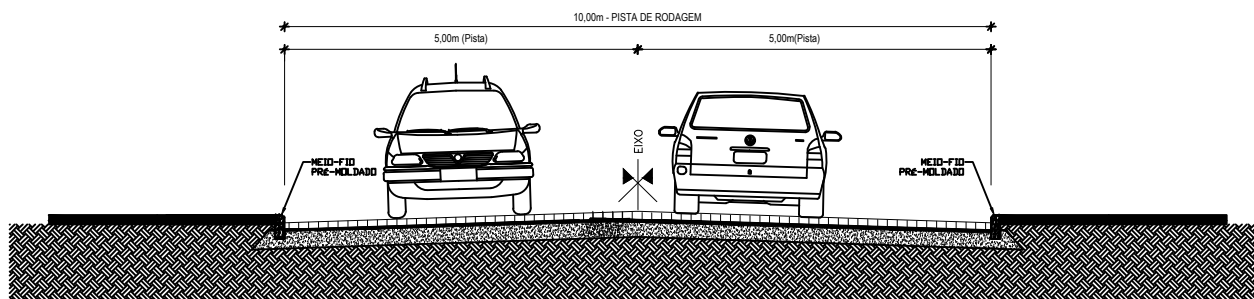
SEÇÃO TIPO DE PAVIMENTAÇÃO COM BLOCO INTERTRAVADO - RUA VEREADOR SELFREDO STEIN
